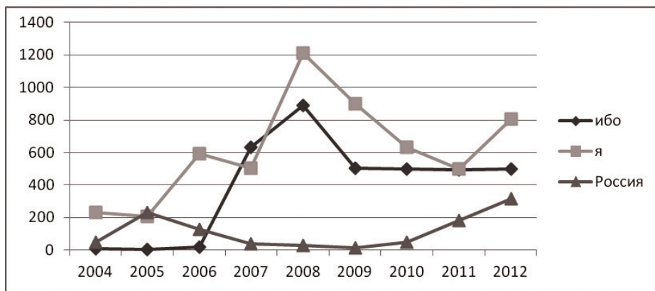
Рисунок 1. Динамика частоты встречаемости отдельных основных категорий (тем) в пророчествах А.Л. Маслова с 2004 по 2012 гг.
